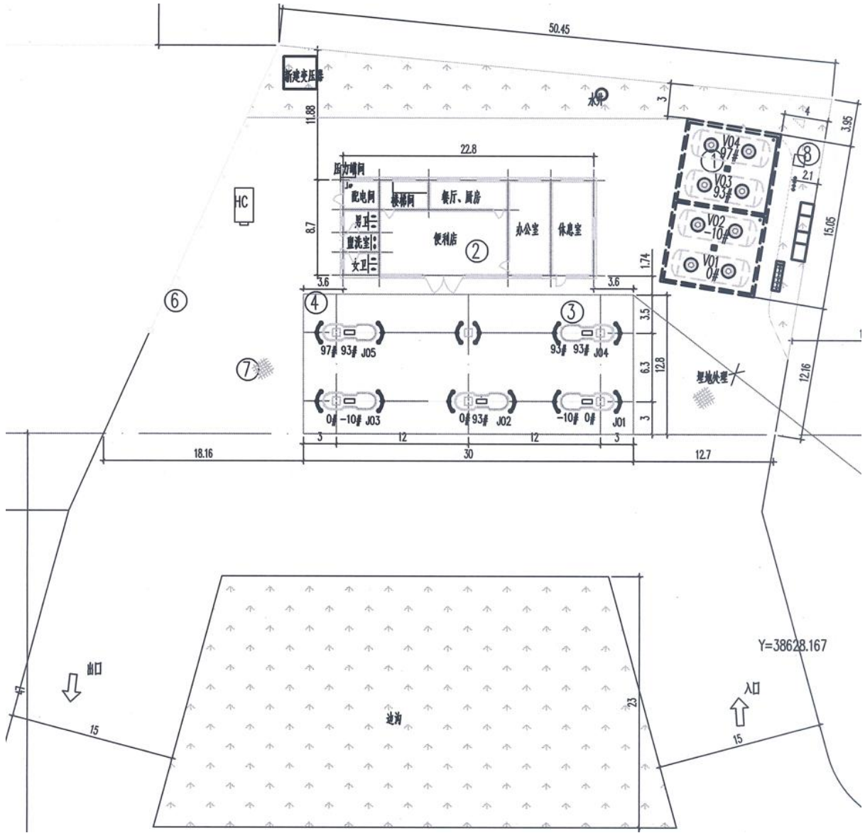
加油站平面图
